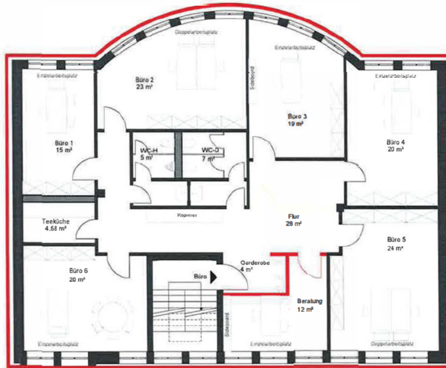
1.Obergeschoss M 1:100
